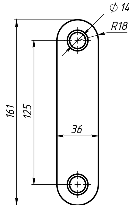
Поз.4 (Серьга)
