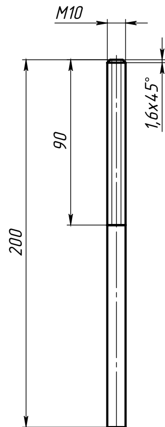
Поз.1 (Шпилька)
